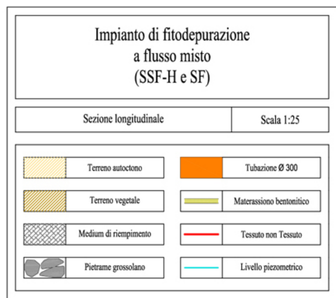
Profilo Idraulico "A-A"
